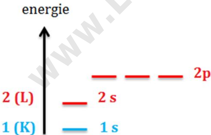
Diagrama energetică pentru primele două straturi electronice
